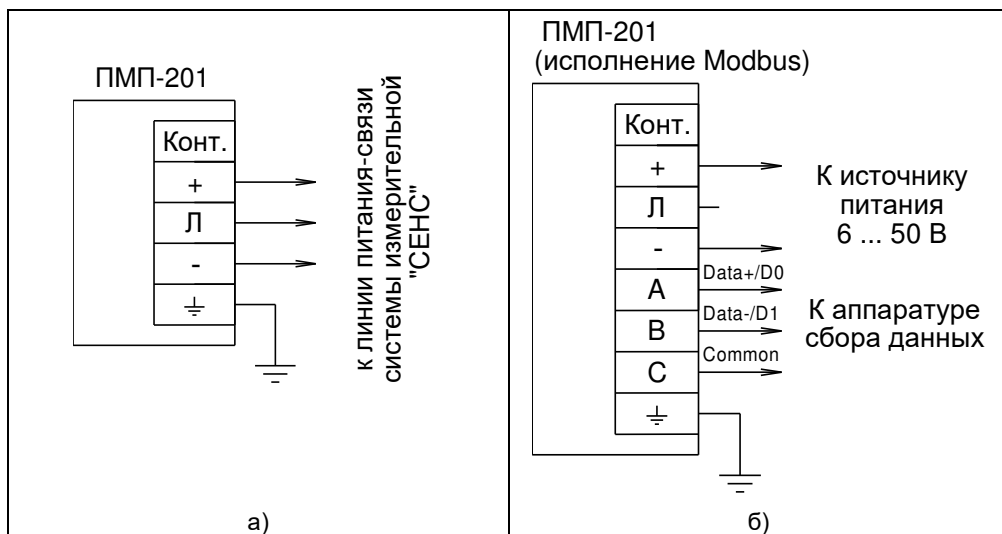
Рисунок 11 – Схема подключения:
