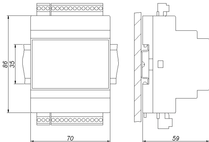
Рисунок 1 – Габаритно-присоединительные размеры модуля
