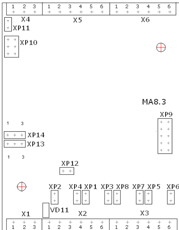
Рисунок 2 - Плата модуля МА8.3
